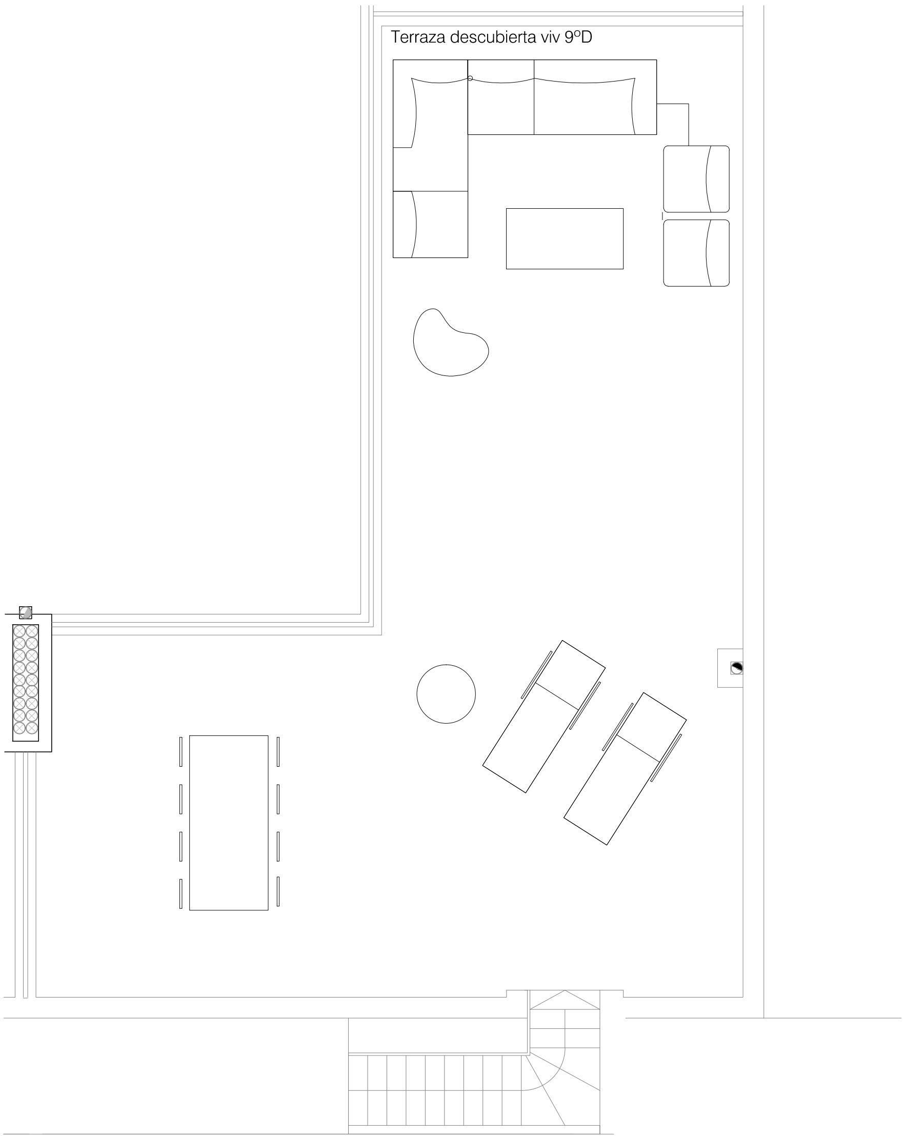
PLANTA CUBIERTA VIVIENDA D TERRAZA DESCUBIERTA 62.15 M2
